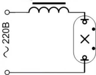
Рис. 2 Схема включения
