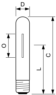
SON-T 400W E E40
