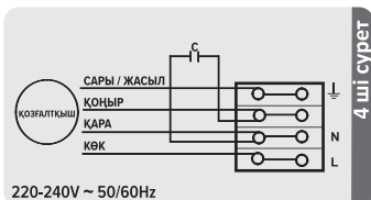
Электрмонтаждық кестесі CYCLONE EBM / TORNADO EBM / MARS GDF
