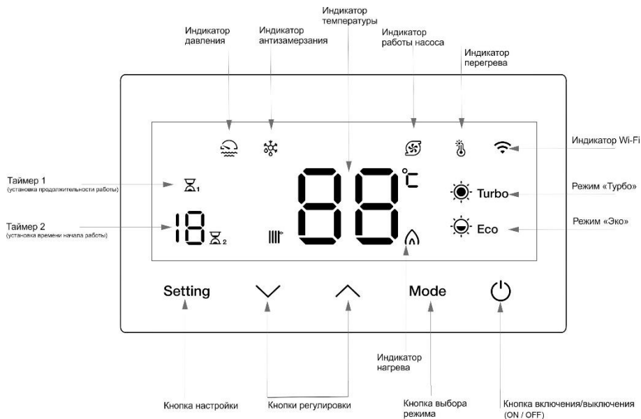
Рис. 3. Панель управления
