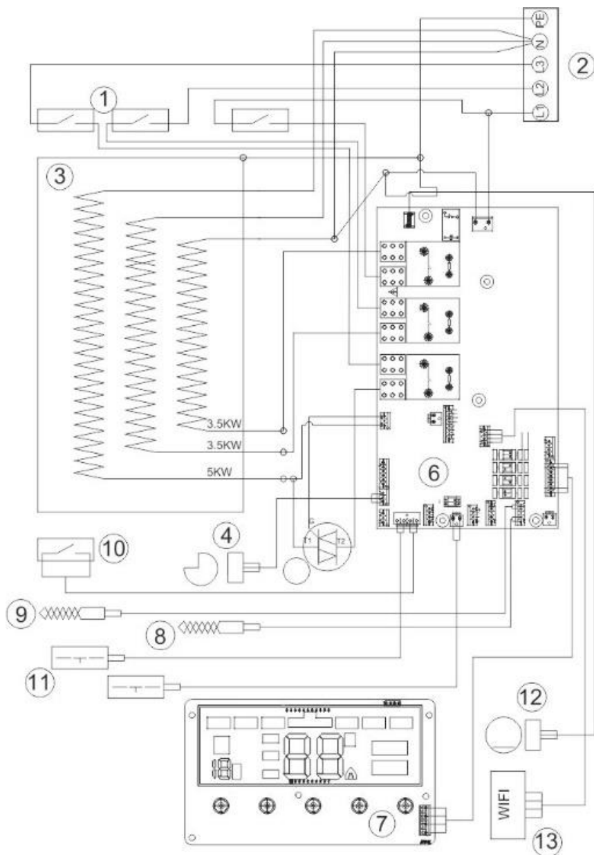
Рис. 15. Электрическая схема THERMEX Grizzly 5-12 Wi-Fi
