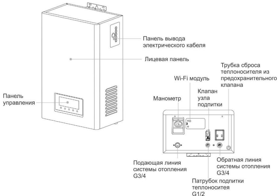
Рис. 1. Конструкция изделия
