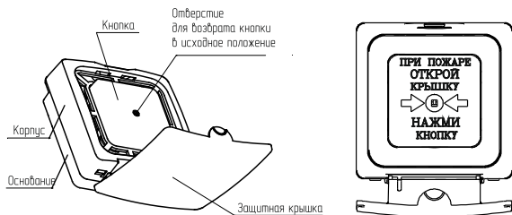
Рисунок 1- Внешний вид и устройство извещателя
