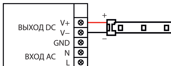
Схема подключения
