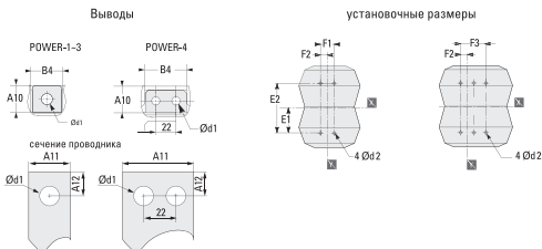
Рис.2 Присоединительные размеры
