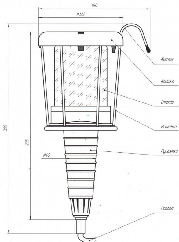
Герметичный светильник НРП
