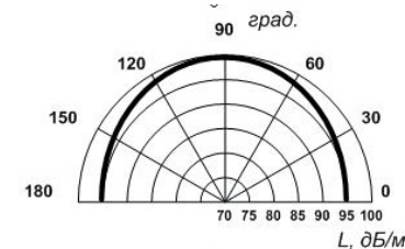
Рисунок 1 – Диаграмма направленности оповещателя
