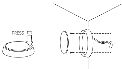
Рис. 1. Монтаж светильника
