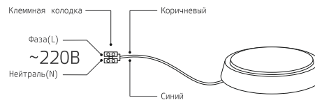
Рис. 2. Схема подключения светильника к электросети 220 В
