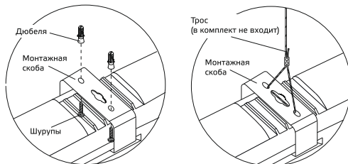
Рис. 4. Схема установки
