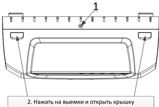
Рисунок 1. Вид сверху
