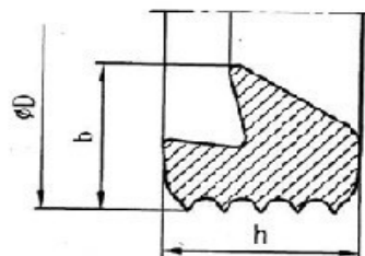
Рисунок 2. Уплотнительного кольца однолепесткового типа.
