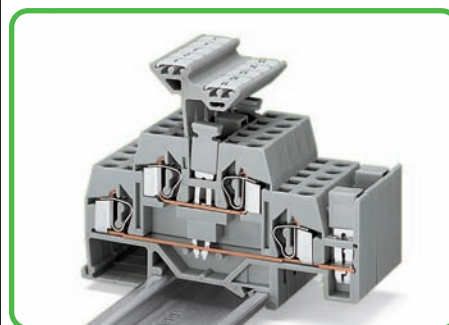
Объединение перемычками двухуровневых клемм
